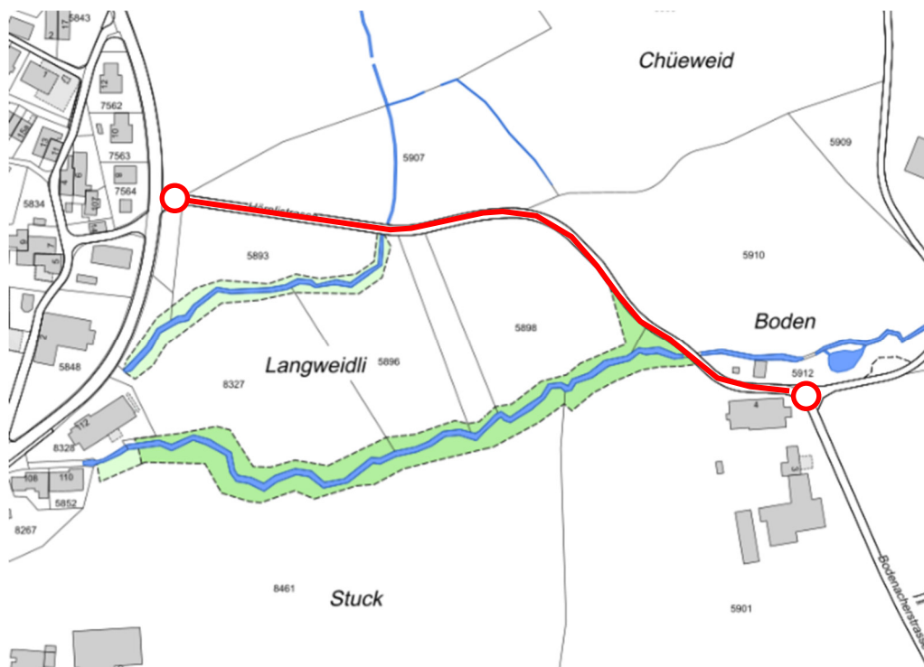
Abbildung 1: Baustellenperimeter
