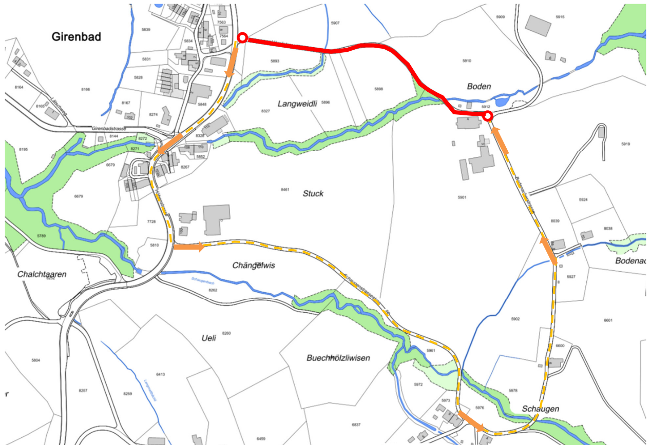
Abbildung 2: Umleitung
